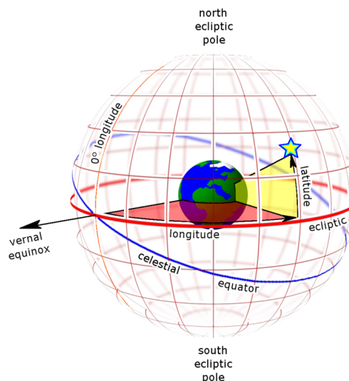
Ảnh 4: Hình minh họa hệ tọa độ hoàng đạo
